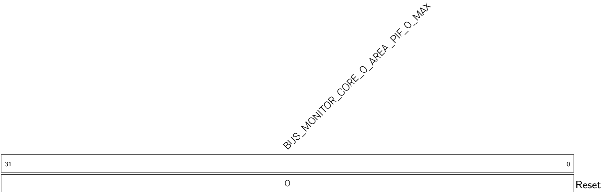
Register 14.22. BUS_MONITOR_CORE_O_AREA_PIF_O_MAX_REG (0x0024)
