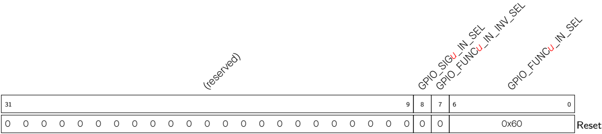
Register 5.20. GPIO_FUNC U _IN_SEL_CFG_REG ( U : 97-116) (0x0448+0x4*( U -97))
