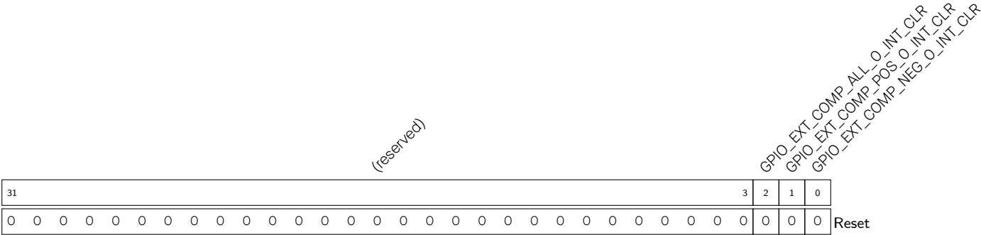
Register 5.40. GPIO_EXT_INT_CLR_REG (0x01DC)
