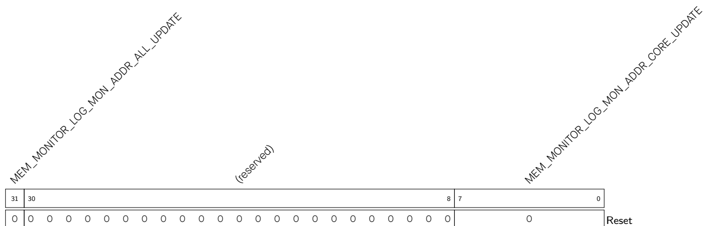
Register 14.7. MEM_MONITOR_LOG_MON_ADDR_UPDATE_0_REG (0x0018)
