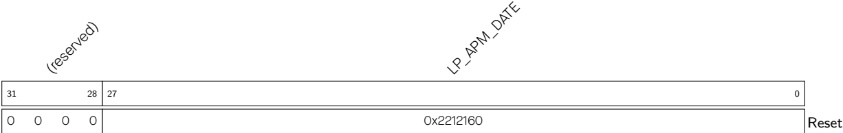
Register 13.44. LP_APM_DATE_REG (0x00FC)
