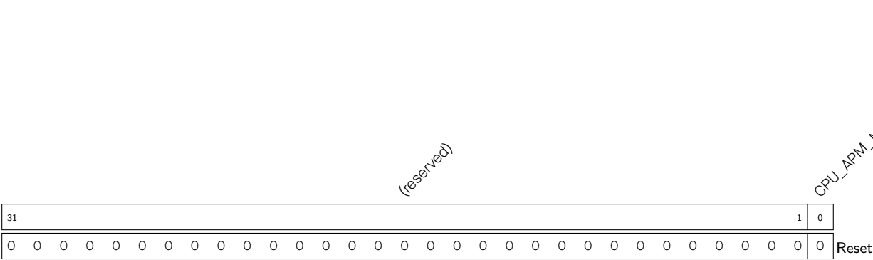
Register 13.63. CPU_APM_MO_STATUS_CLR_REG (0x00CC)
