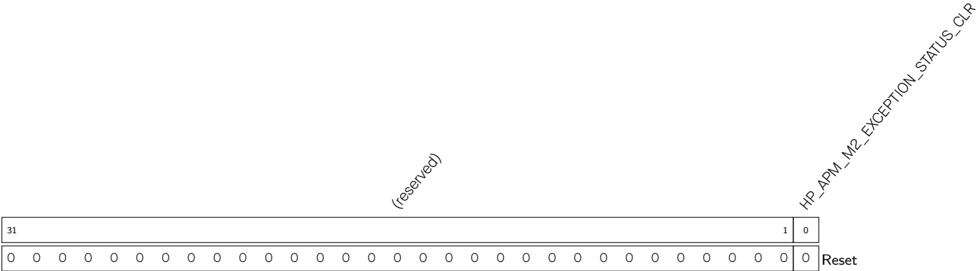
Register 13.15. HP_APM_M2_STATUS_CLR_REG (0x00EC)
