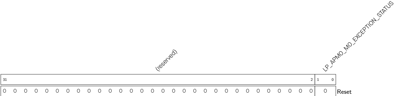
Register 13.50. LP_APMO_MO_STATUS_REG (0x00C8)
