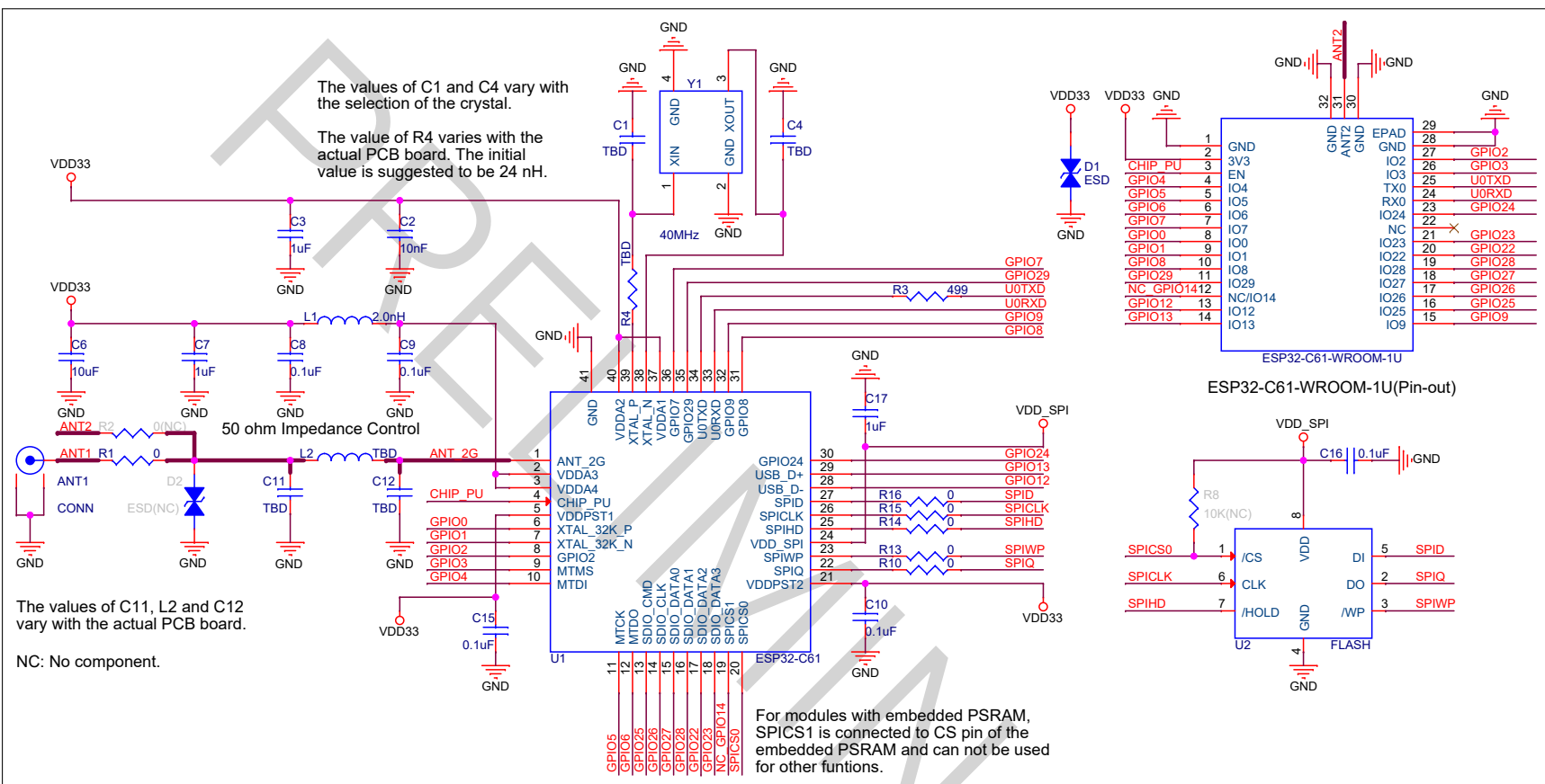
图 7: ESP32-C61-WROOM-1U 原理图
