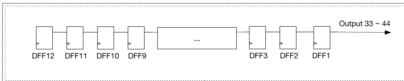
图 4.3-3. 移位寄存器电路图 (后 12 字节)
