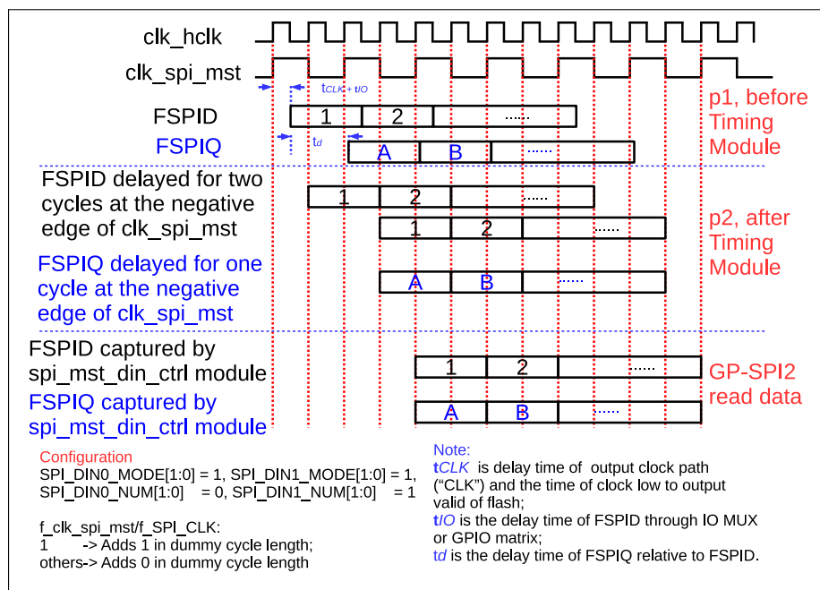
图 23.8-2. GP-SPI2 主机时序补偿示例
