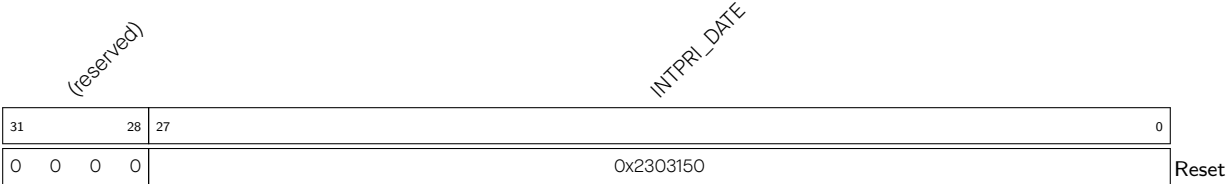
Register 7.54. INTPRI_DATE_REG (0x00A0)
