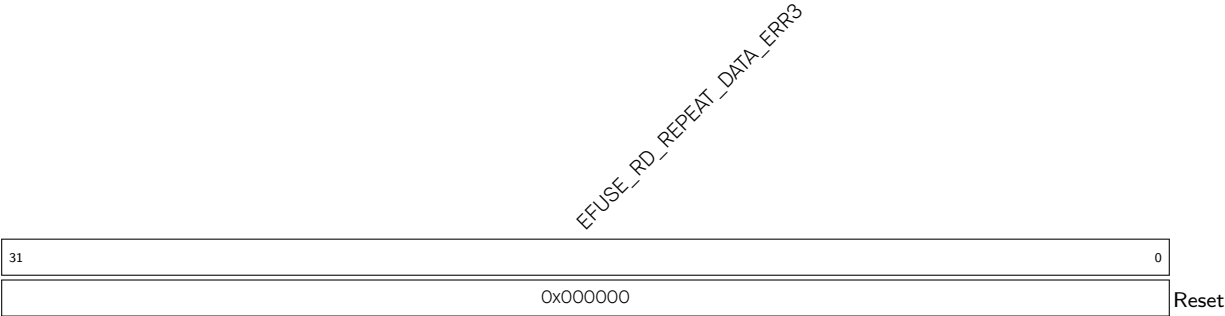
Register 4.27. EFUSE_RD_REPEAT_DATA_ERR3_REG (0x0188)
