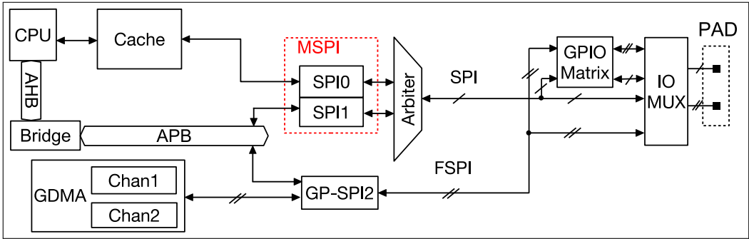
图 23.4-1. SPI 模块概览
