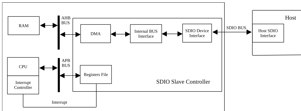
图 27.3-1. SDIO 从机功能结构图
