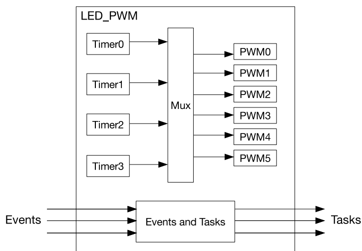
图 28.3-1. LED PWM 控制器架构
