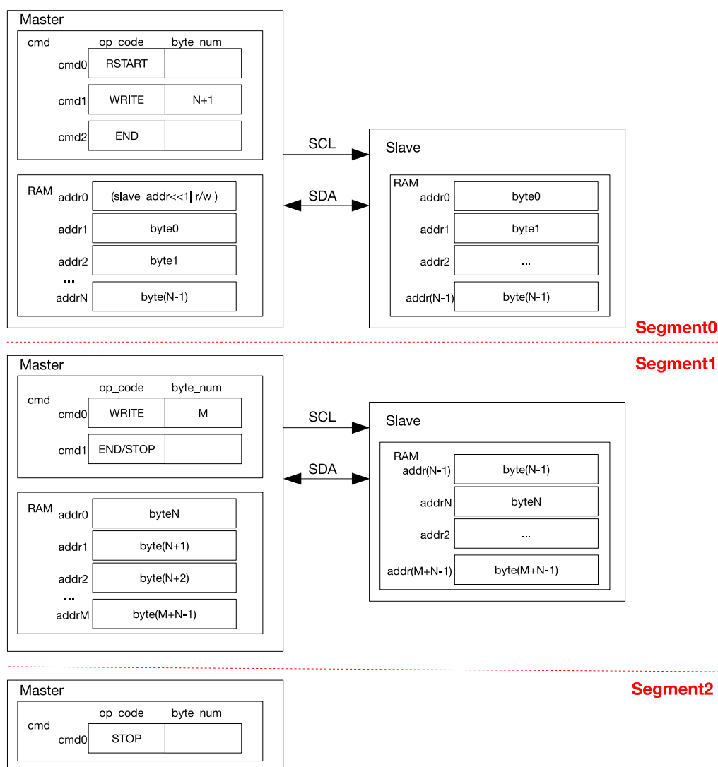
图 24.6-4. I2C 主机分段写 7 位寻址的从机
