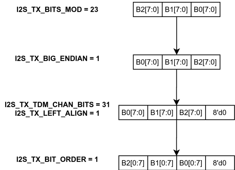
图 25.9-1. TX 数据格式控制
