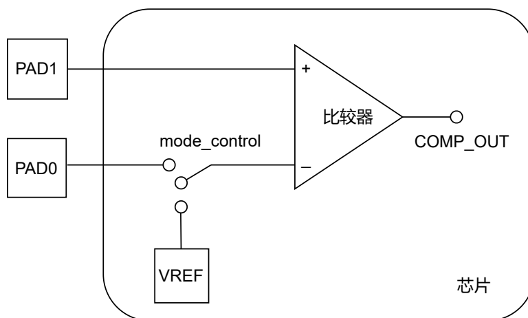
图 31.3-1. 模拟电压比较器系统框图
