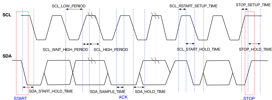
图 24.4-1. I2C 时序图
