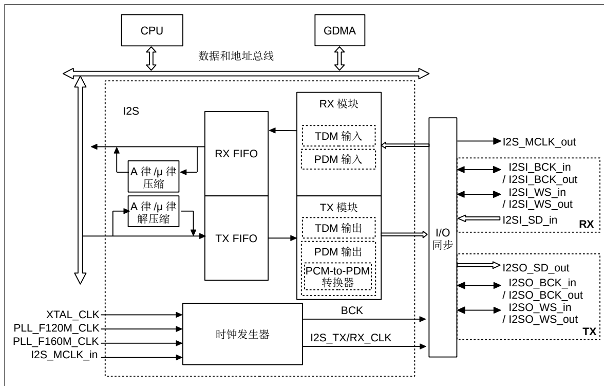
图 25.4-1. ESP32-C61 I2S 系统框图
