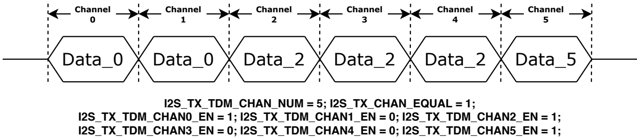
图 25.9-2. TDM 通道控制
