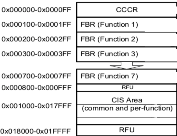
图 27.5-3. function 0 地址空间
