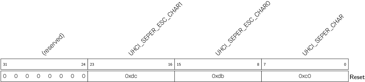
Register 22.58. UHCI_ESC_CONFO_REG (0x006C)
