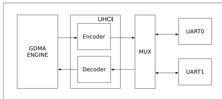
图 22.4-10. GDMA 模式数据传输
