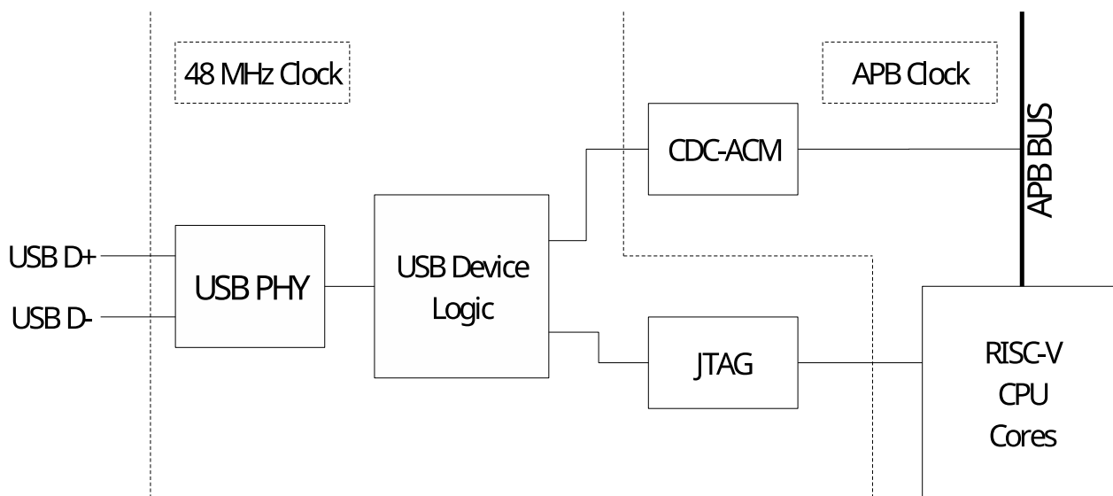
图 26.2-1. USB 串口/JTAG 控制器高层框图
