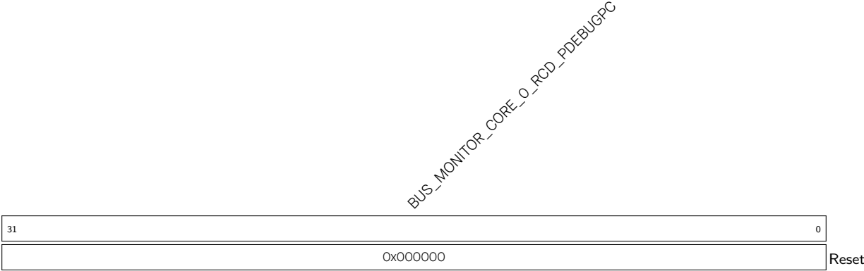
Register 15.34. BUS_MONITOR_CORE_O_RCD_PDEBUGPC_REG (0x0048)
