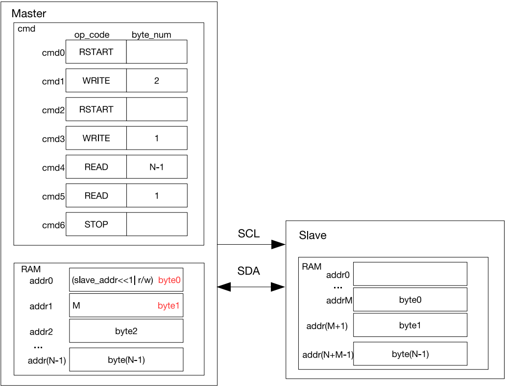
图 24.6-7. I2C 主机从 7 位寻址从机的 M 地址读取 N 个数据
