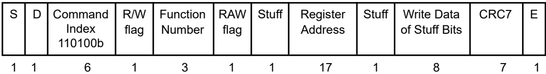
图 27.5-1. CMD52 内容
