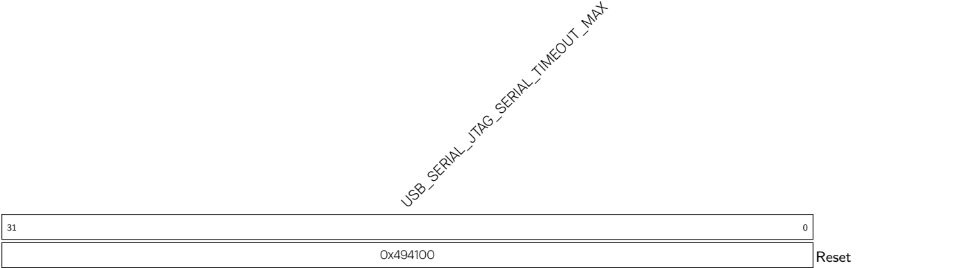
Register 26.13. USB_SERIAL_JTAG_SERIAL_EP_TIMEOUT1_REG (0x0070)
