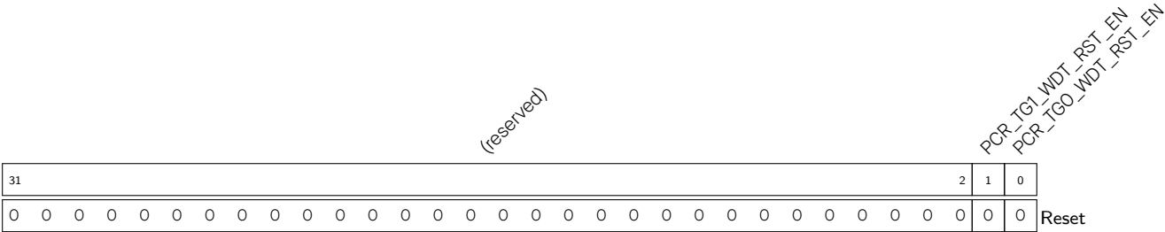
Register 5.64. PCR_TIMERGROUP_WDT_CONF_REG (0x012C)
