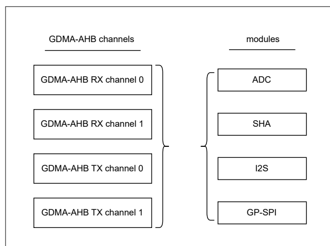
图 2.1-1. 共用 GDMA 通道的模块
