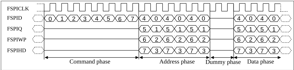
图 23.5-8. GP-SPI2 发送到 Flash 的 SPI Quad I/O 命令序列
