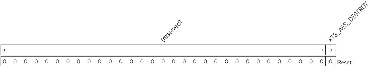
Register 20.9. XTS_AES_DESTROY_REG (0x0354)
