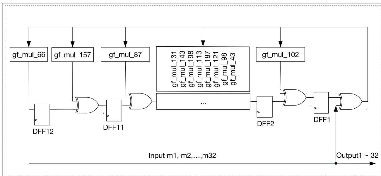
图 4.3-2. 移位寄存器电路图 (前 32 字节)
