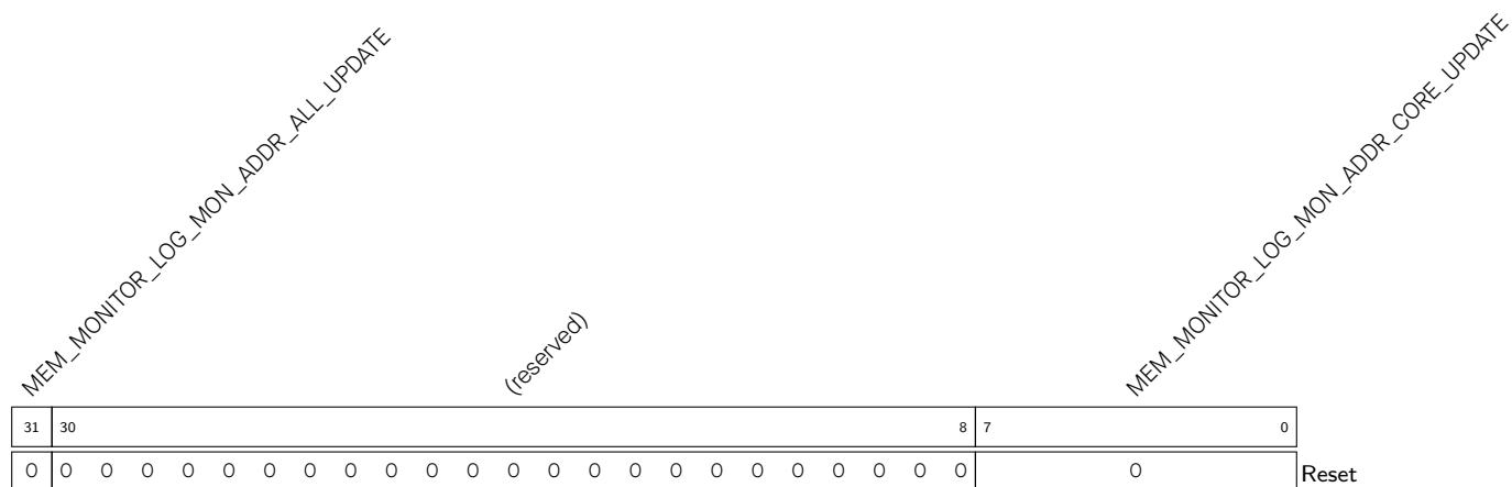
Register 15.7. MEM_MONITOR_LOG_MON_ADDR_UPDATE_0_REG (0x0018)
