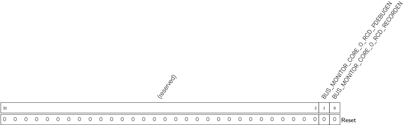
Register 15.33. BUS_MONITOR_CORE_O_RCD_EN_REG (0x0044)
