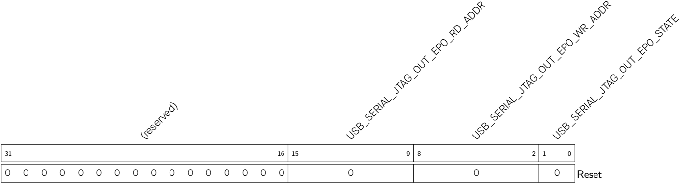
Register 26.24. USB_SERIAL_JTAG_OUT_EPO_ST_REG (0x0038)
