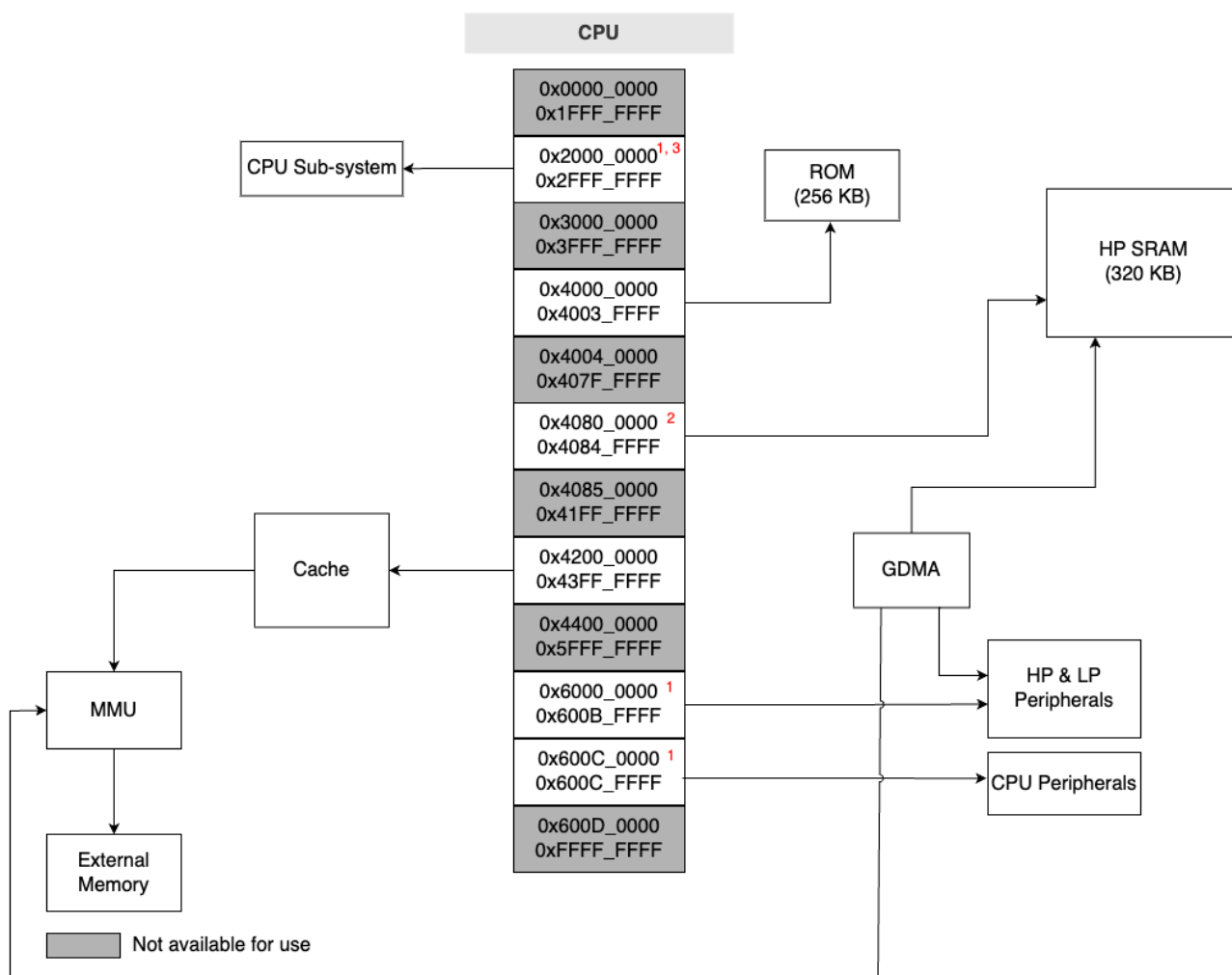
图 3.3-1. 系统结构与地址映射结构
