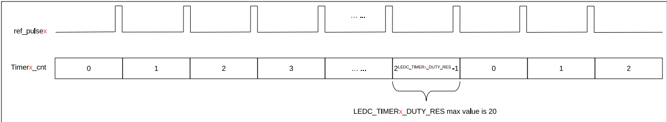
图 28.4-2. 计数器和 PWM 信号精度关系
