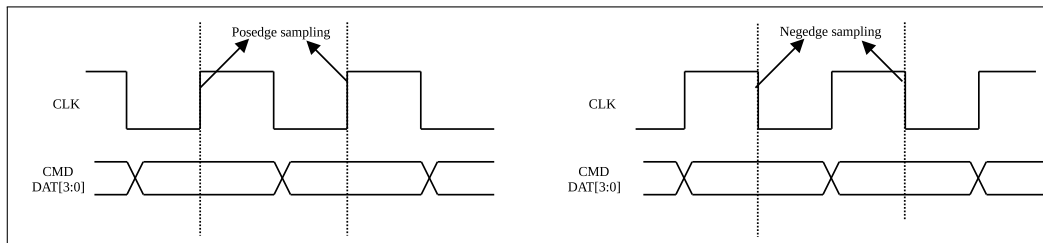
图 27.5-8. 采样时序图
