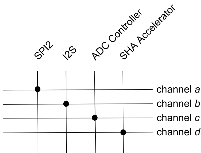
图 3.3-3. 具有 GDMA 功能的外设/模块
