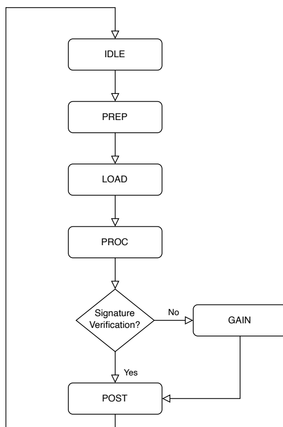
图 19.5-1. ECDSA 流程
