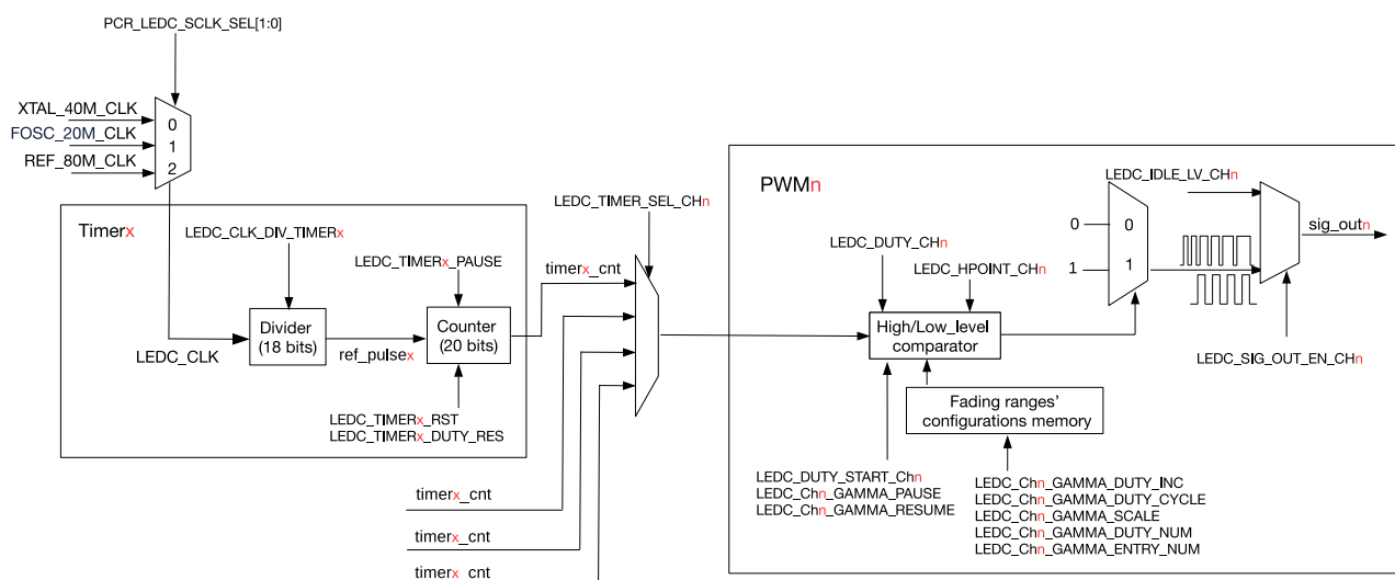
图 28.3-2. 定时器和 PWM 生成器功能框图
