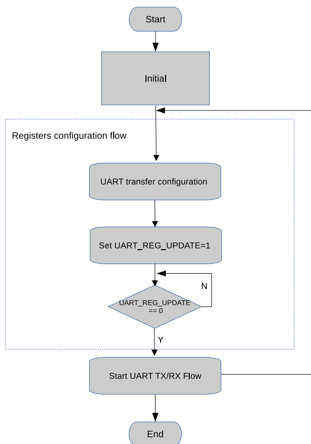
图 22.6-1. UART 编程流程
