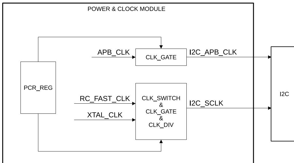
图 5.3-1. I2C 时钟配置示例
