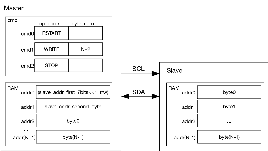
图 24.6-2. I2C 主机写 10 位寻址的从机
