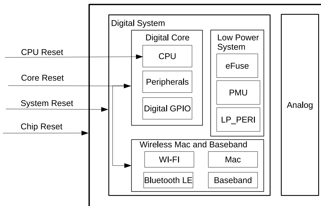
图 5.1-1. 四种复位等级
