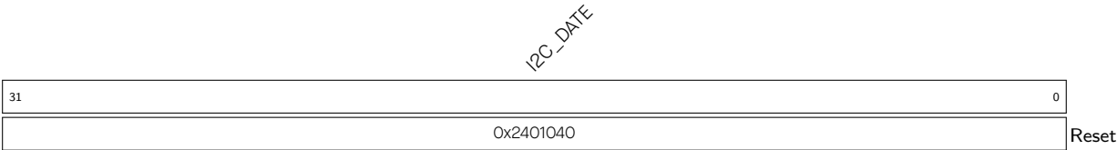
Register 24.33. I2C_DATE_REG (0x00F8)
