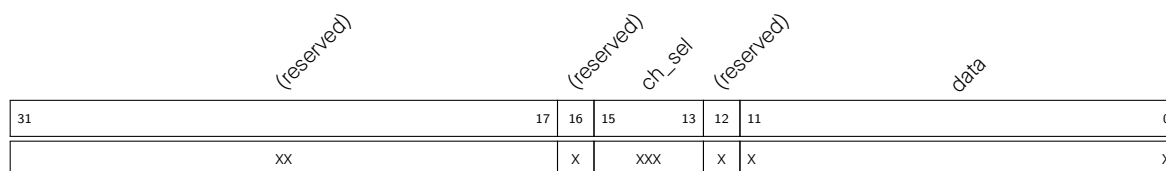
图 30.5-8. GDMA 数据格式
