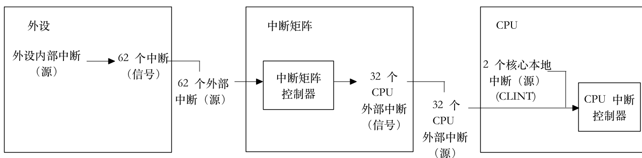
图 7.2-1. ESP32-C61 的中断流
