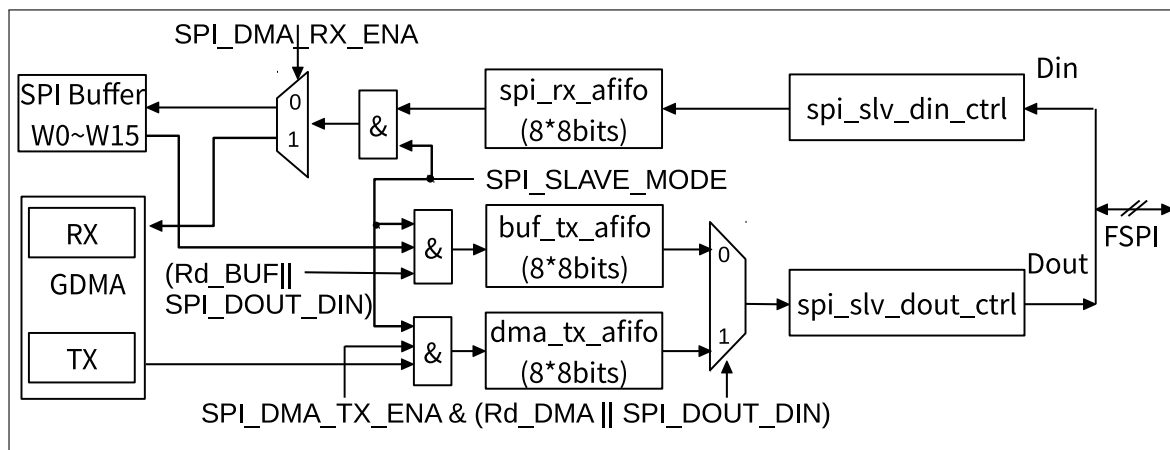
图 23.5-4. GP-SPI2 用作从机时的数据流控制
