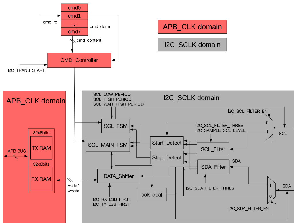
图 24.3-1. I2C 主机基本架构
