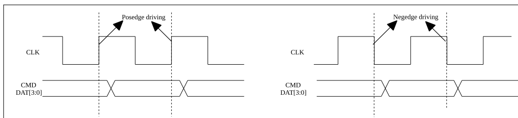
图 27.5-9. 输出时序图
