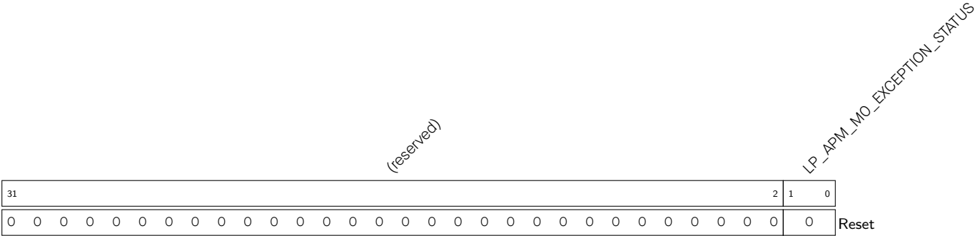
Register 14.30. LP_APM_MO_STATUS_REG (0x00C8)
