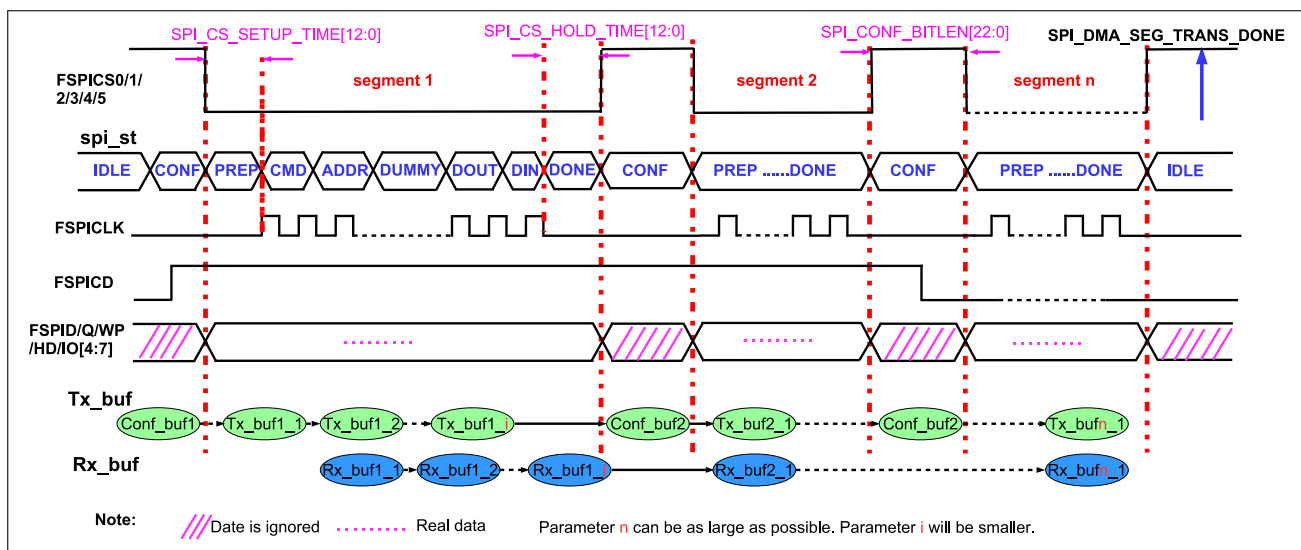
图 23.5-9. DMA 控制的分段配置传输
