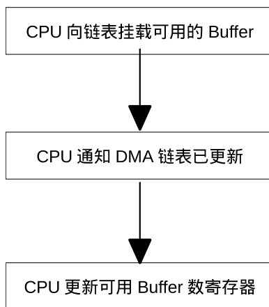
图 27.7-3. 从机 CPU 挂载 buffer 的流程
