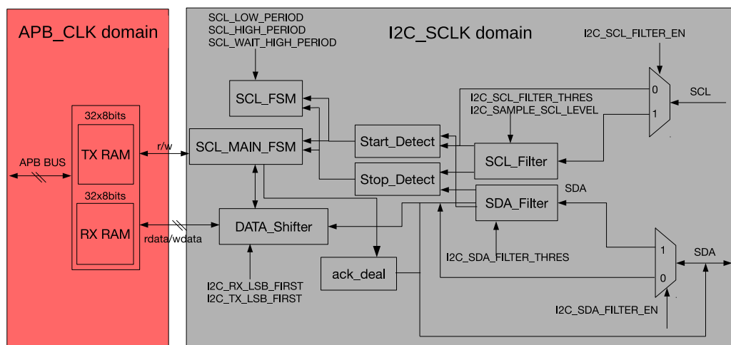
图 24.3-2. I2C 从机基本架构
