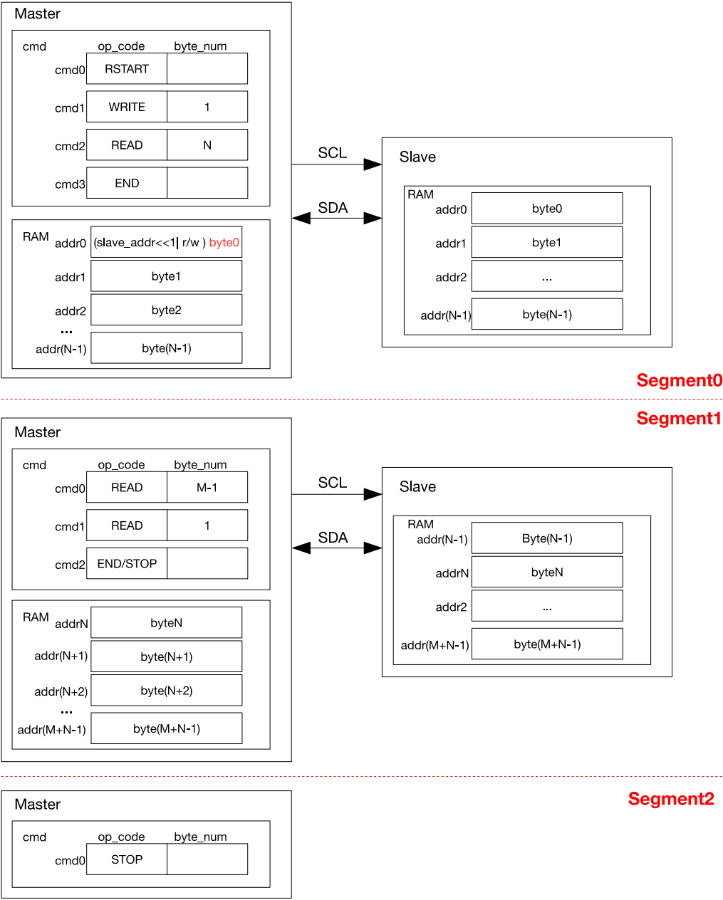
图 24.6-8. I2C 主机分段读 7 位寻址的从机
