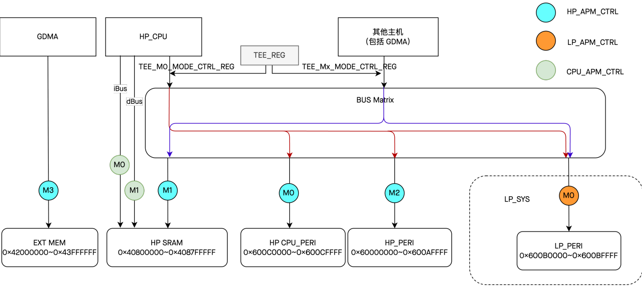
图 14.5-1. APM 控制器结构图
