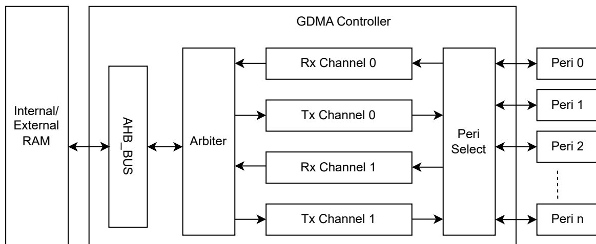
图 2.3-1. GDMA 控制器的架构
