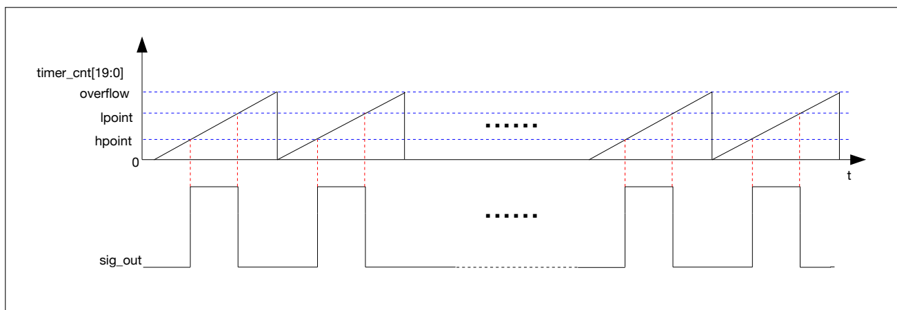
图 28.4-3. LED PWM 输出信号图
