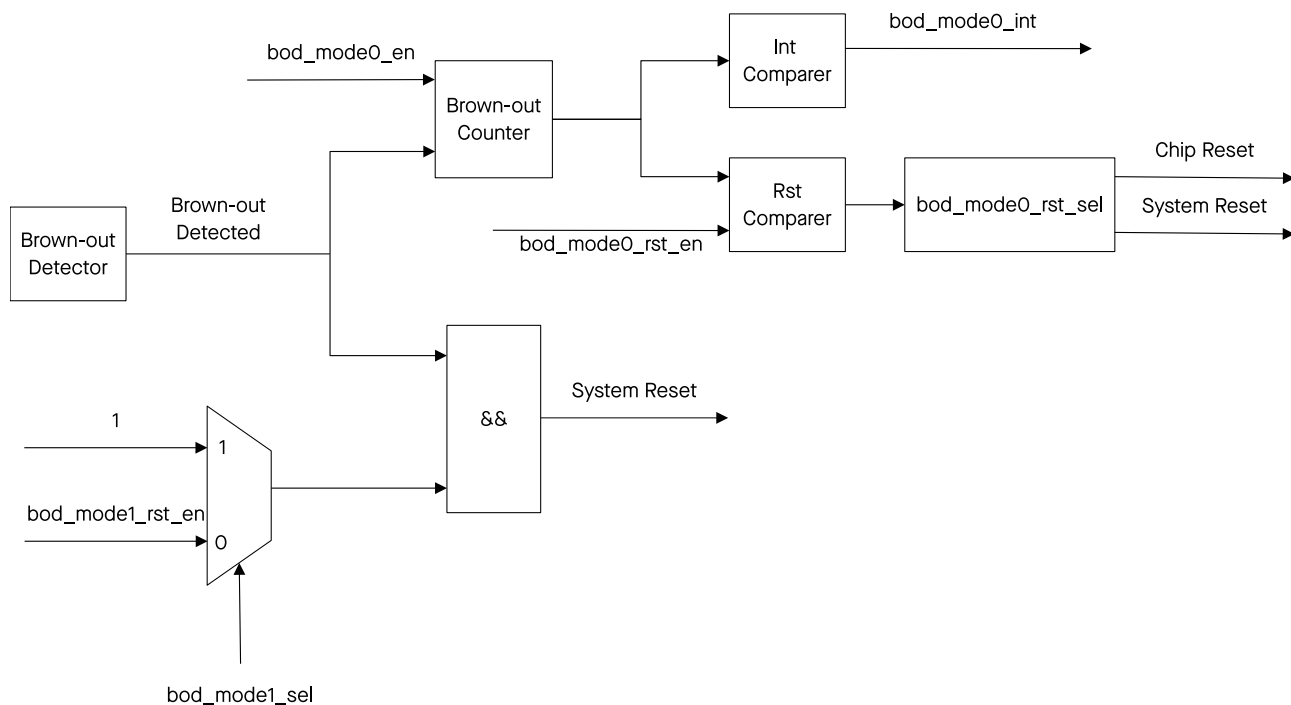
图 16.3-2. 欠压检测器处理方式
