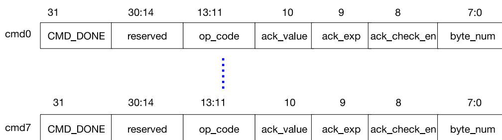
图 24.4-2. I2C 命令寄存器结构
