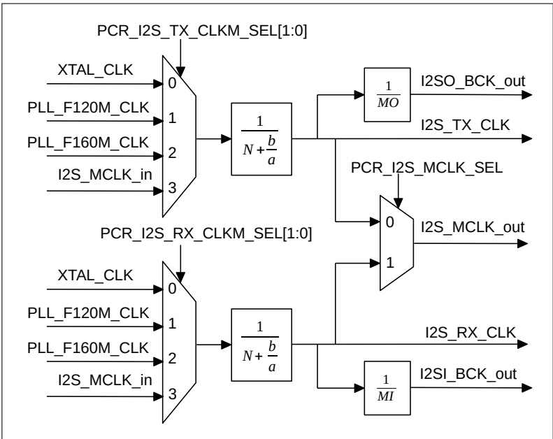
图 25.6-1. I2S 时钟分频器
