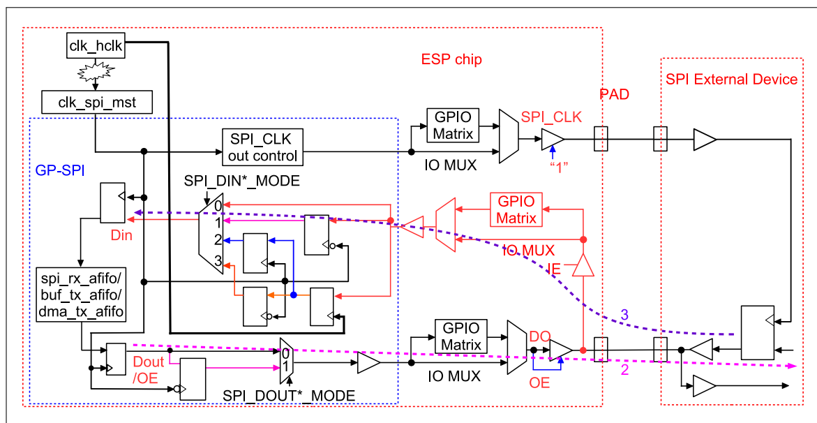
图 23.8-1. GP-SPI2 主机时序补偿控制图
