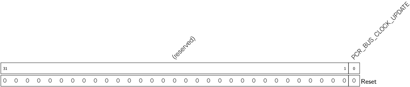
Register 5.62. PCR_BUS_CLK_UPDATE_REG (0x0120)
