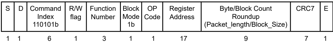
图 27.5-2. CMD53 内容
