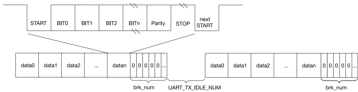
图 22.4-3. UART 数据帧结构
