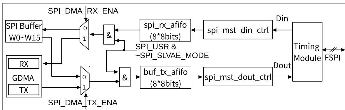
图 23.5-3. GP-SPI2 用作主机时的数据流控制
