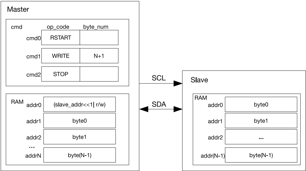
图 24.6-1. I2C 主机写 7 位寻址的从机
