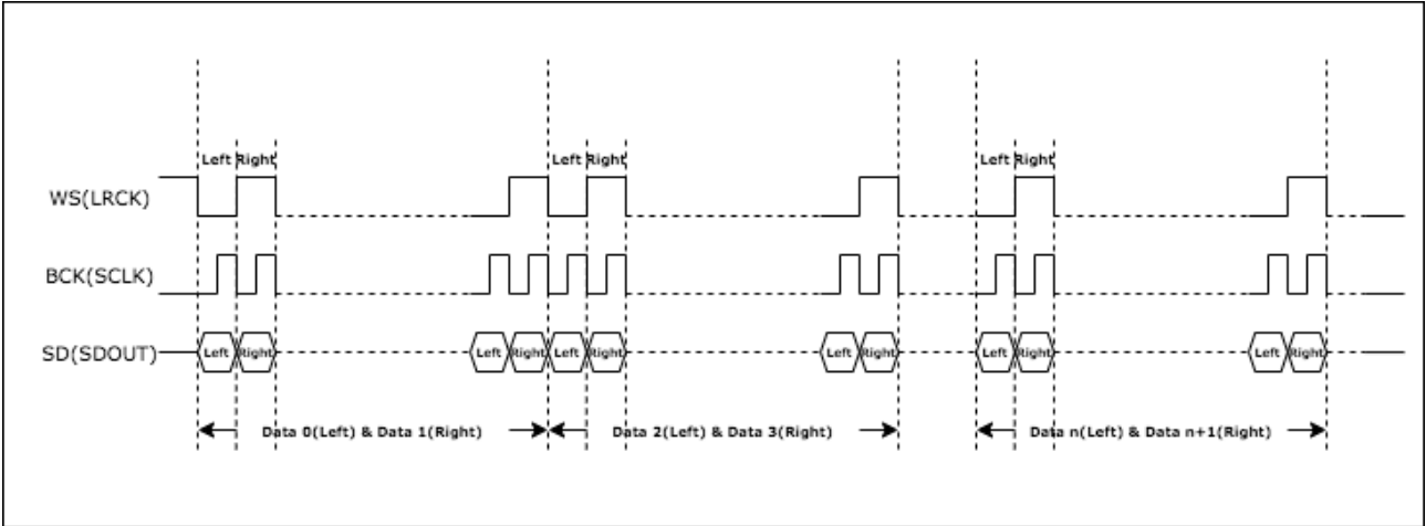
图 25.5-4. 时序图 – PDM 标准
