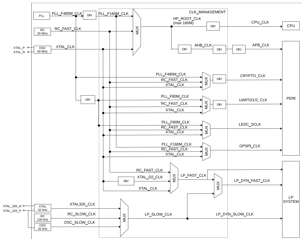
图 5.2-1. 系统时钟
