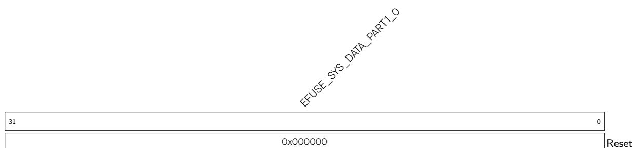
Register 4.15. EFUSE_RD_SYS_PART1_DATA n _REG ( n : 0-7) (0x005C+0x4* n )
