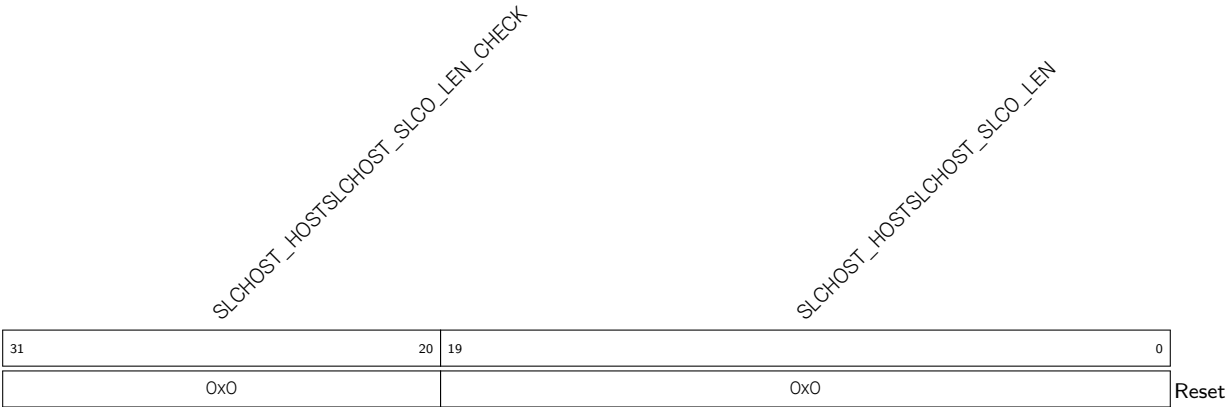
Register 27.51. SLCHOST_PKT_LEN_REG (0x0060)
