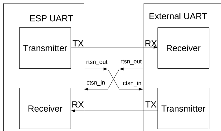
图 22.4-9. 硬件流控信号连接图
