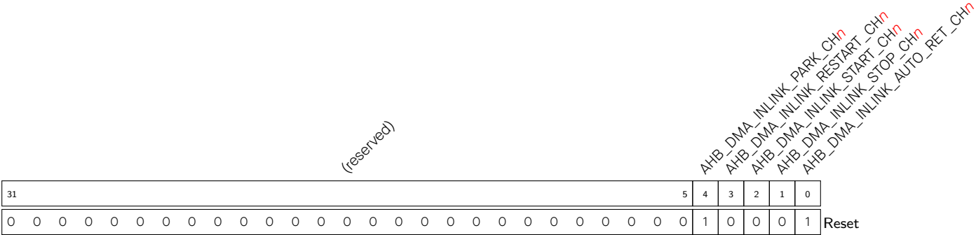
Register 2.13. AHB_DMA_IN_LINK_CHn_REG (n: 0-1) (0x0080+0xC0*n)
