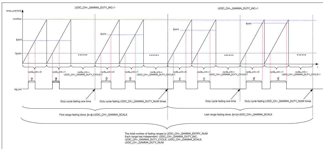
图 28.4-5. 输出信号占空比伽马曲线渐变图
