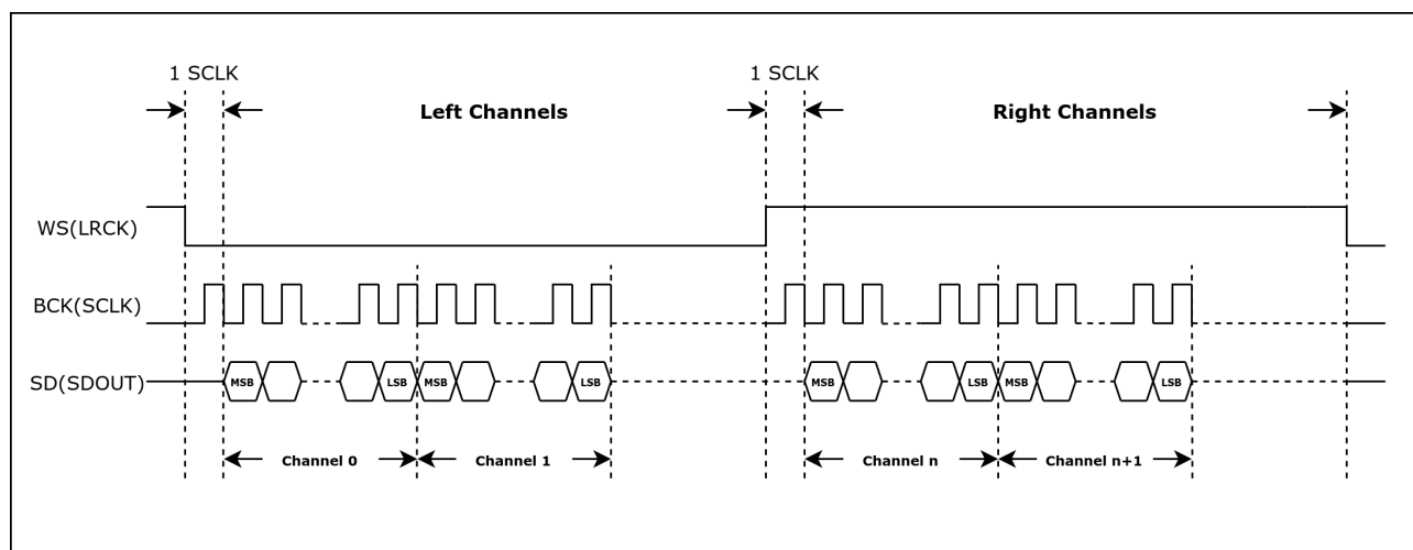
图 25.5-1. 时序图 – TDM Philips 标准
