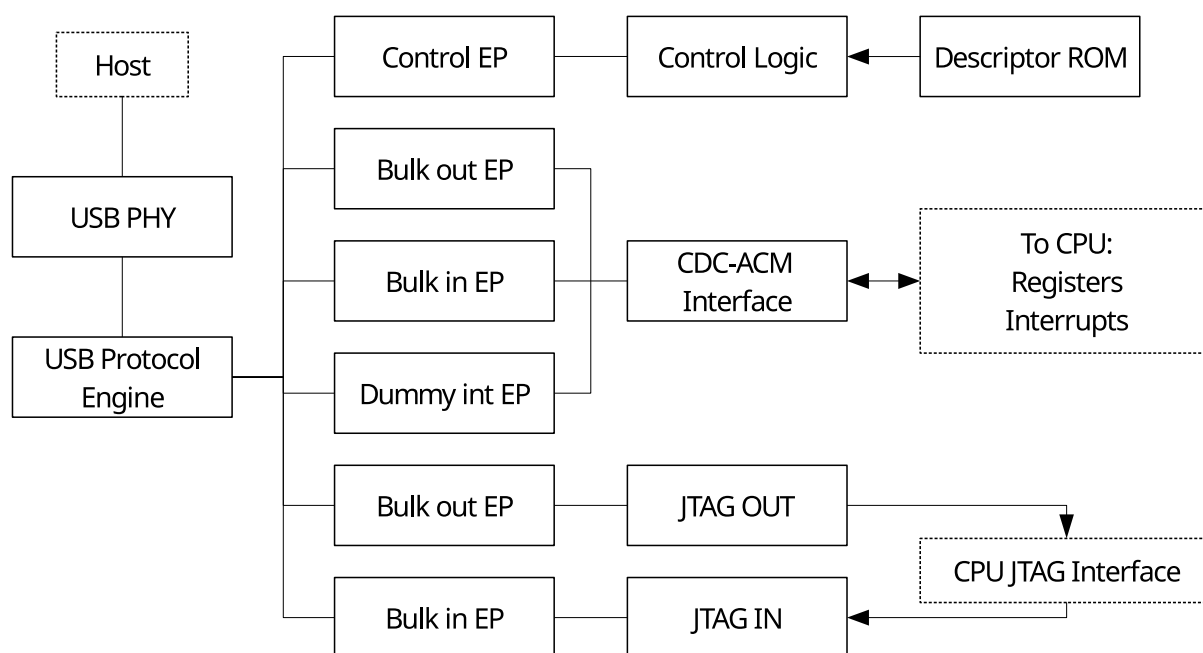
图 26.2-2. USB 串口/JTAG 控制器框图
