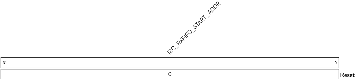
Register 24.35. I2C_RXFIFO_START_ADDR_REG (0x0180)
