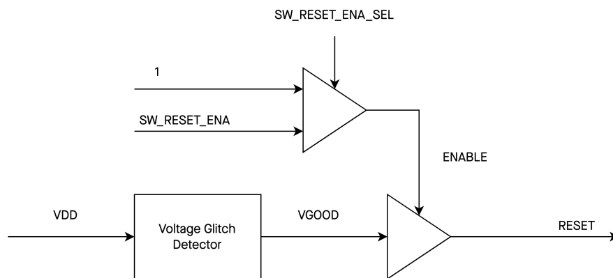
图 16.3-3. 电压毛刺检测器
