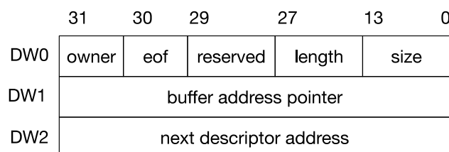
图 27.5-5. SDIO 从机 DMA 链表描述符结构
