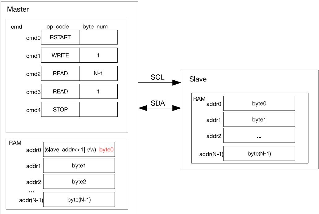
图 24.6-5. I2C 主机读 7 位寻址的从机
