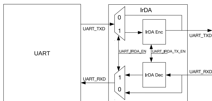
图 22.4-7. IrDA 编解码结构图
