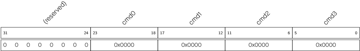
图 30.5-3. APB_SARADC_SAR_PATT_TAB1_REG 包含样式 0 - 3
