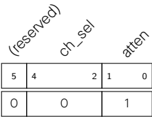
图 30.5-6. cmd0 配置示例
