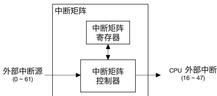
图 7.4-1. 中断矩阵结构图
