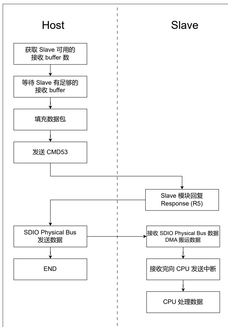
图 27.7-2. 从机从主机接收包的流程
