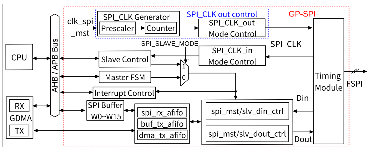
图 23.5-2. GP-SPI2 功能块图
