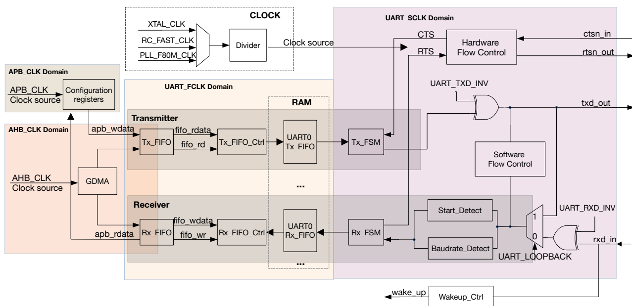
图 22.3-1. UART 基本架构图
