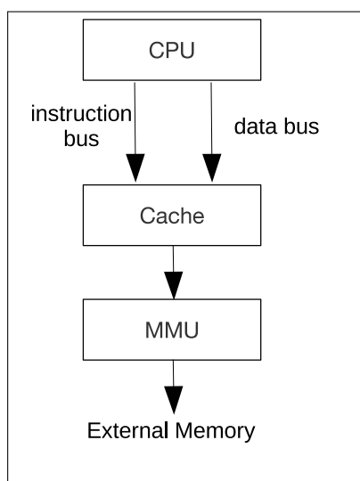
图 3.3-2. Cache 系统结构
