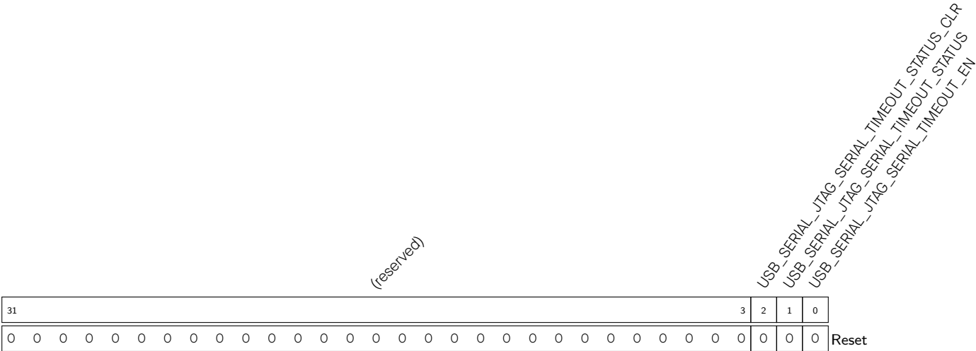
Register 26.12. USB_SERIAL_JTAG_SERIAL_EP_TIMEOUT0_REG (0x006C)
