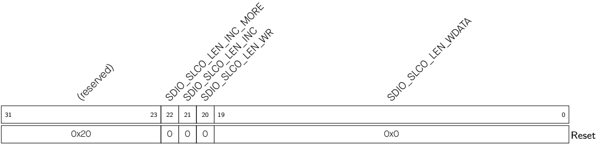
Register 27.20. SDIO_SLCO_LEN_CONF_REG (0x00F4)
