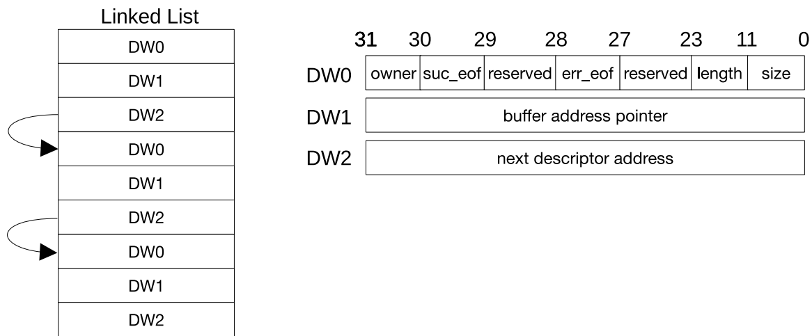
图 2.4-1. 链表结构图
