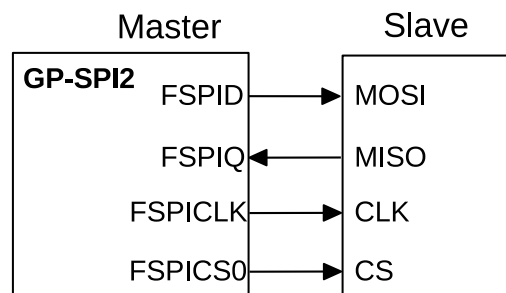
图 23.5-6. GP-SPI2 主机使用全双工模式与 SPI 从机通信框图
