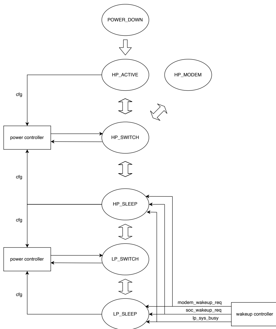
图 9.4-2. PMU 的主要工作流程
