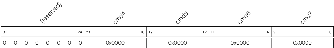
图 30.5-4. APB_SARADC_SAR_PATT_TAB2_REG 包含样式 4 - 7
