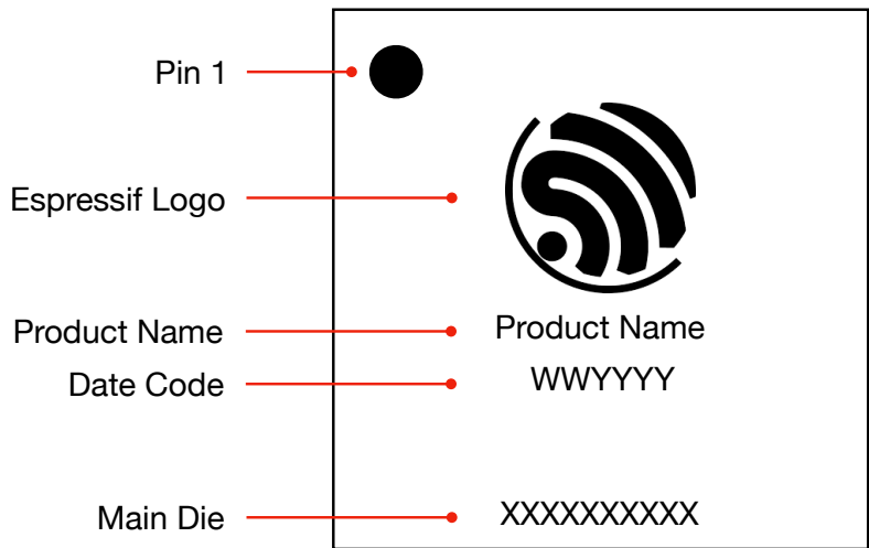
图 1: 芯片丝印示意图
